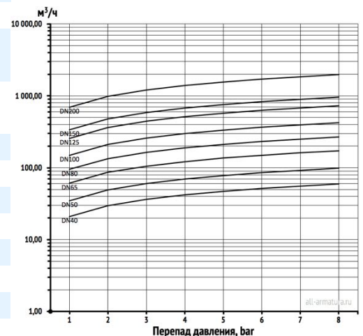
Расходная характеристика
